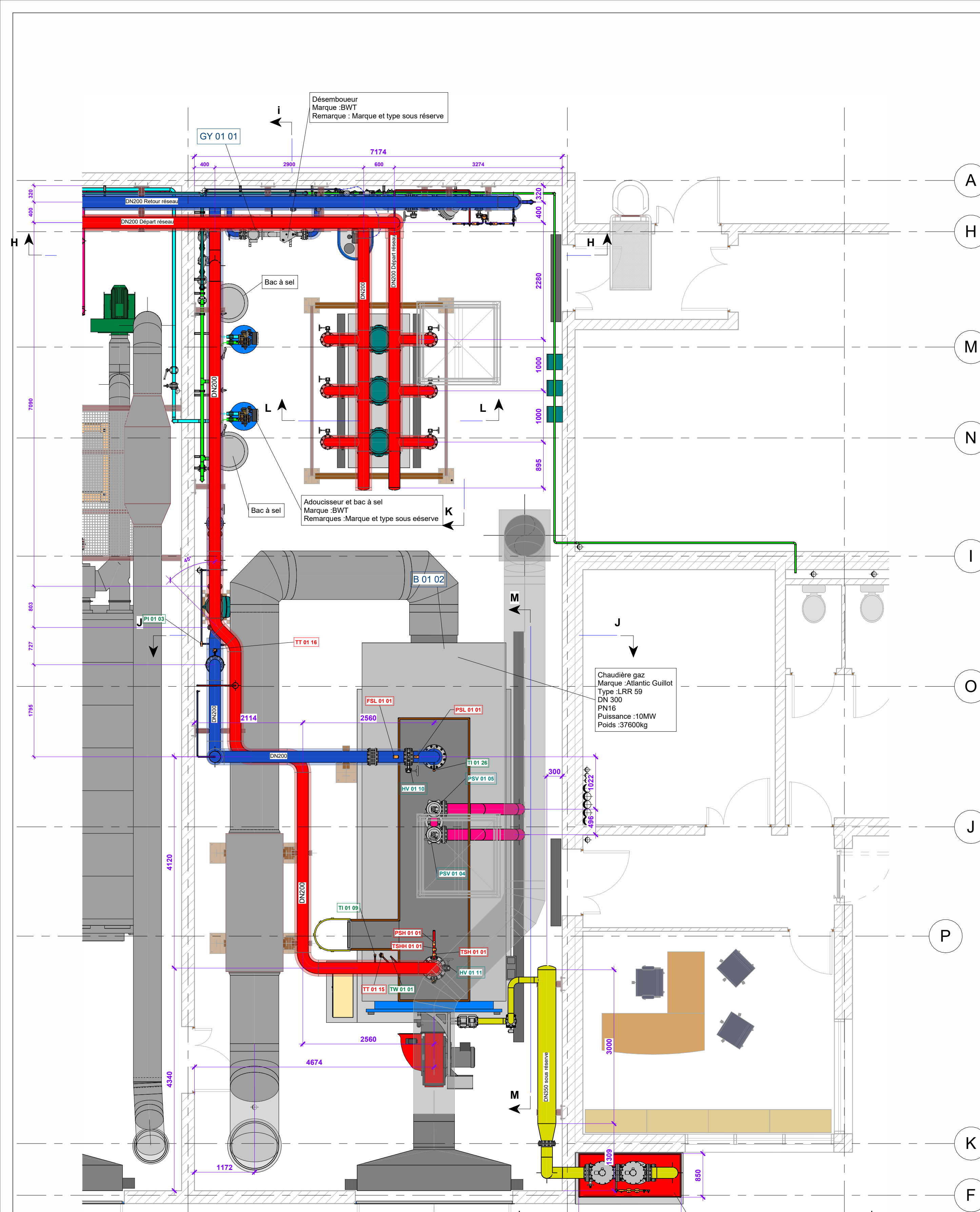
Chaudière gaz Ech : 1 : 50
