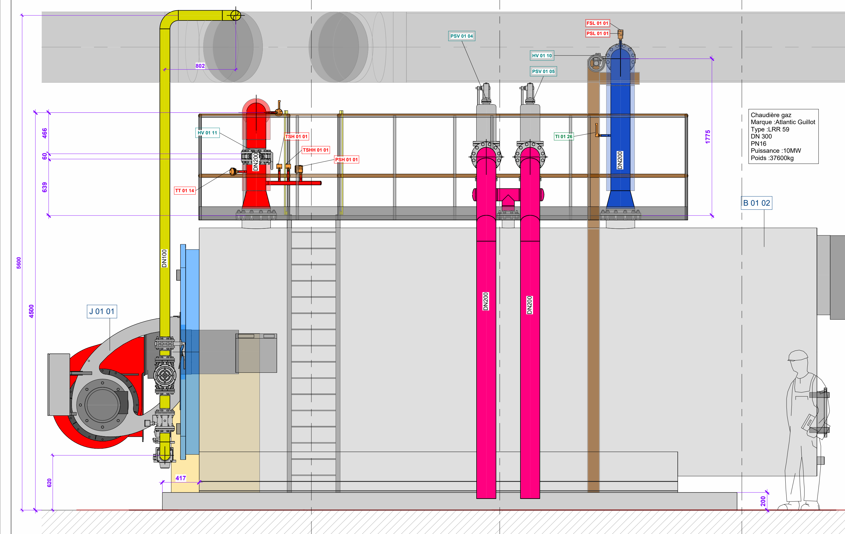
Coupe MM Ech : 1 : 25
