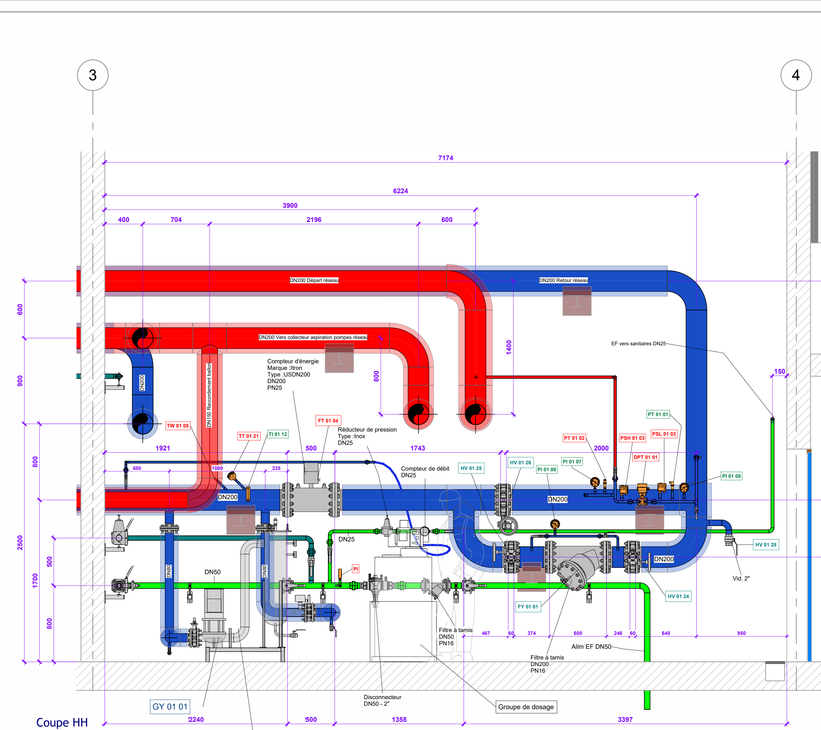
Coupe HH Ech : 1 : 25
