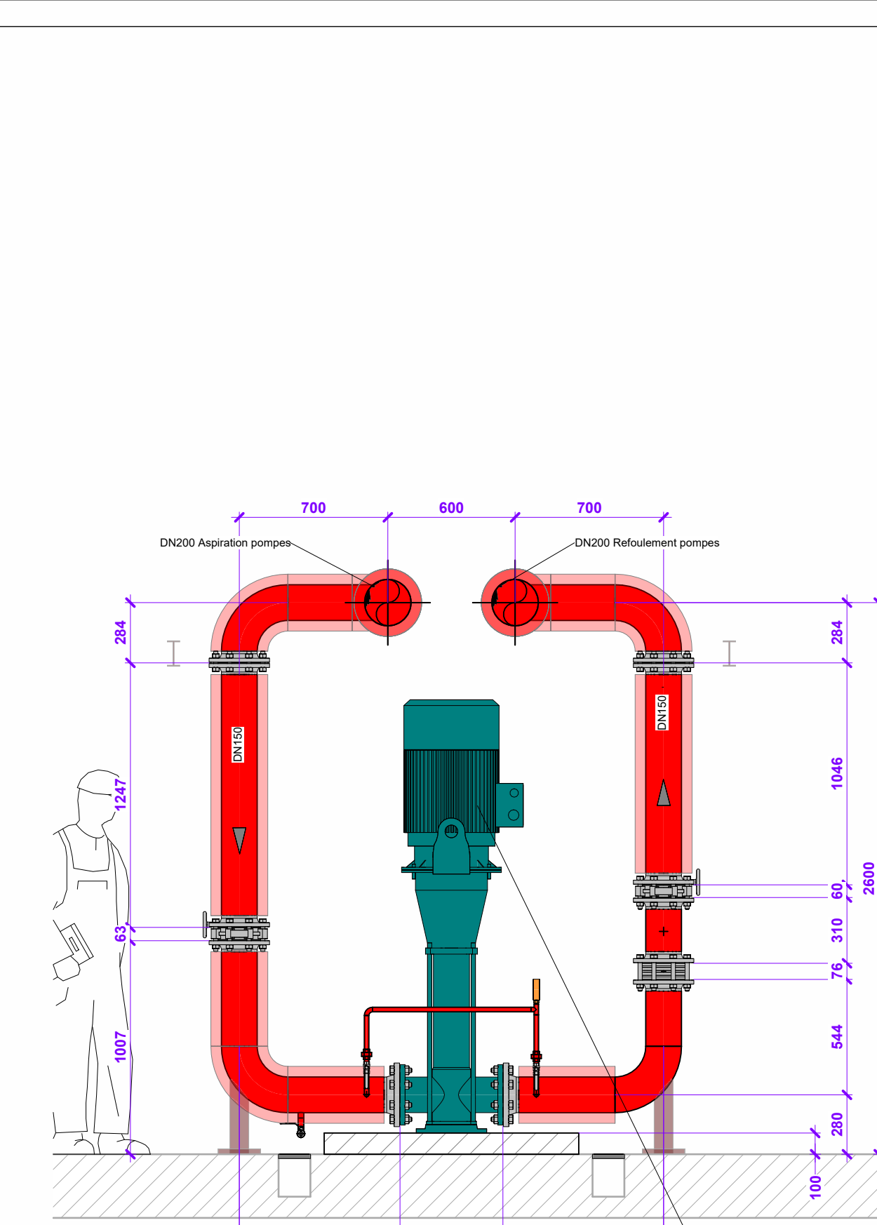
Coupe LL Ech : 1 : 25
