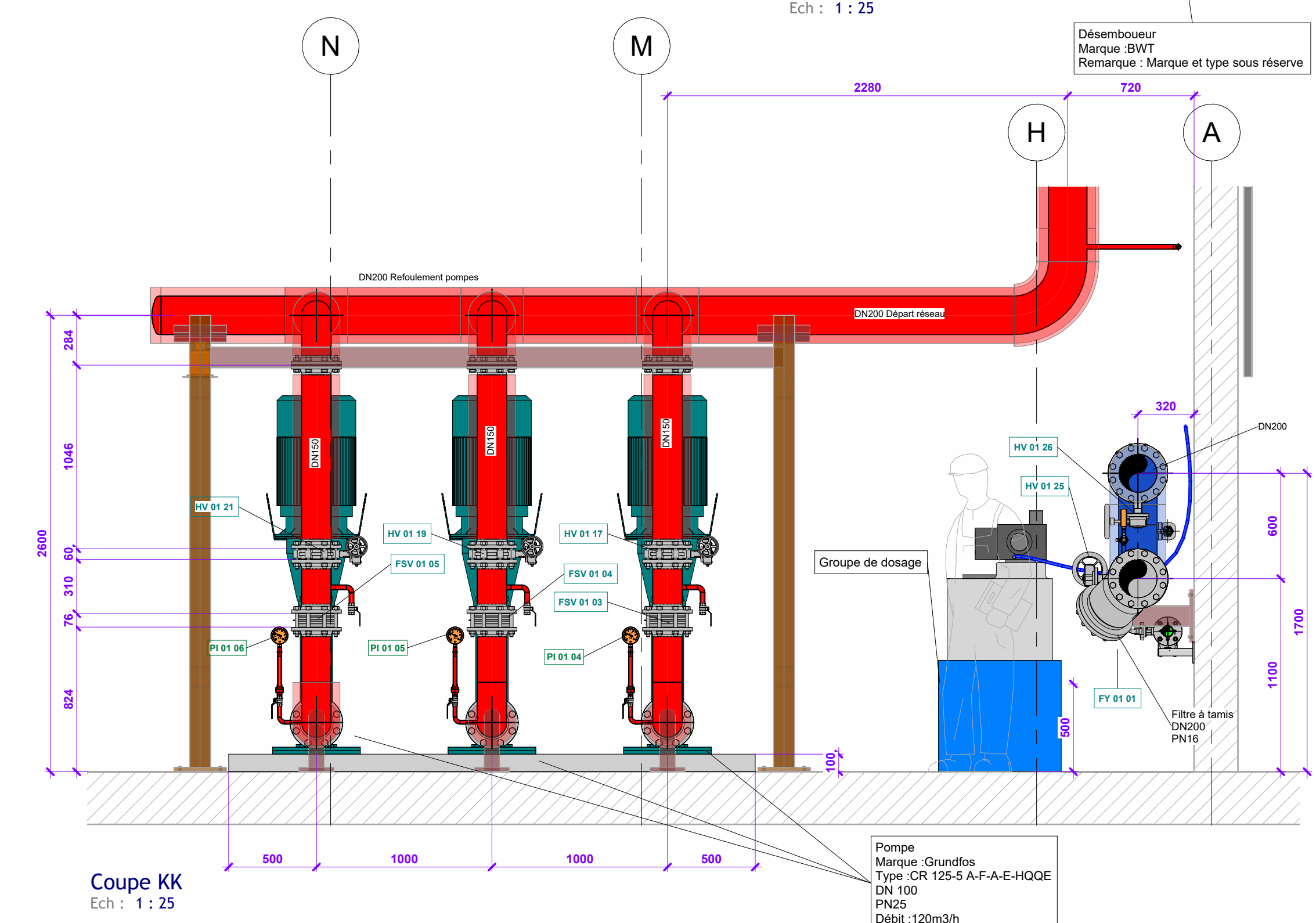
Coupe KK Ech : 1 : 25
