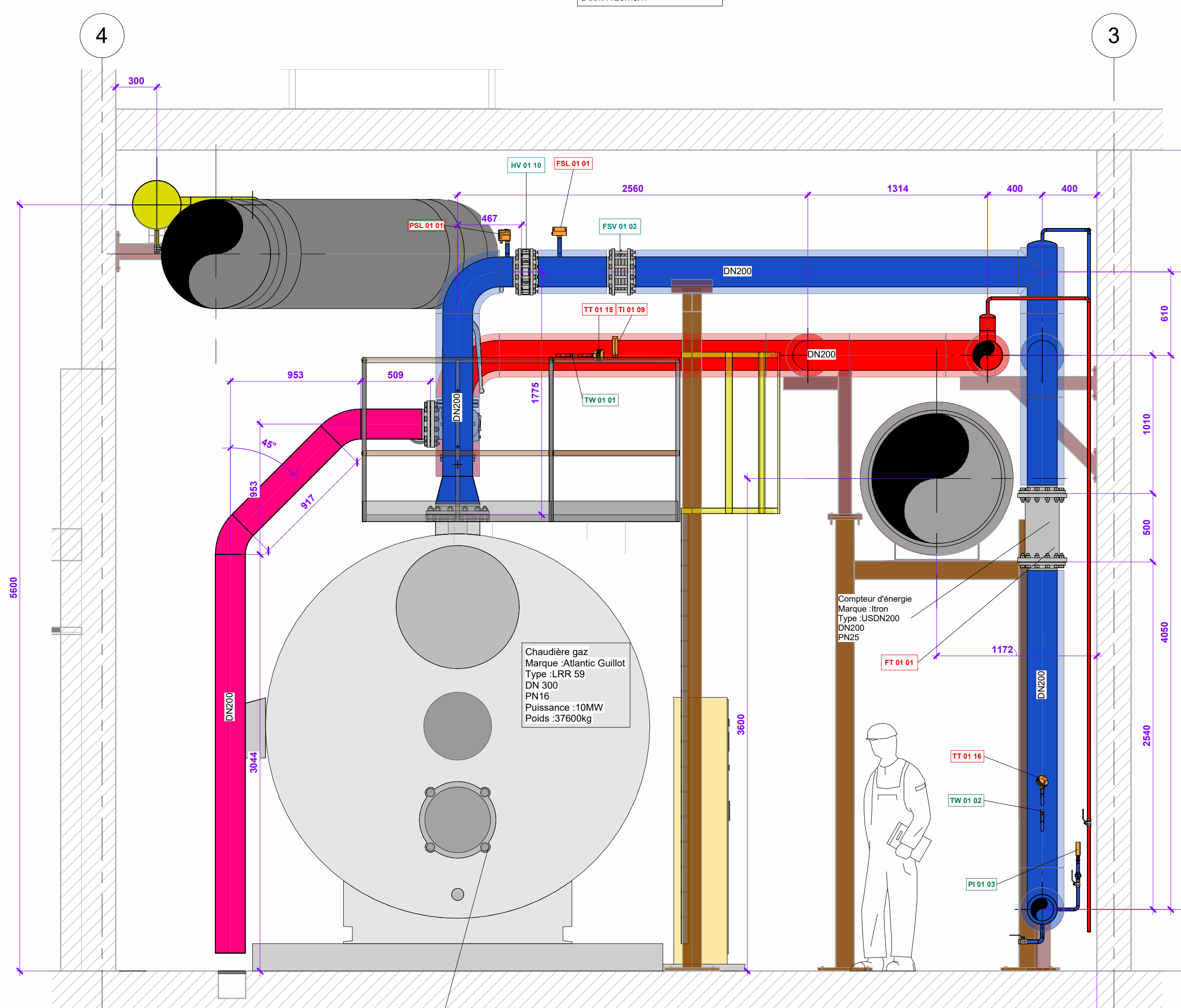
Coupe JJ Ech : 1 : 25
